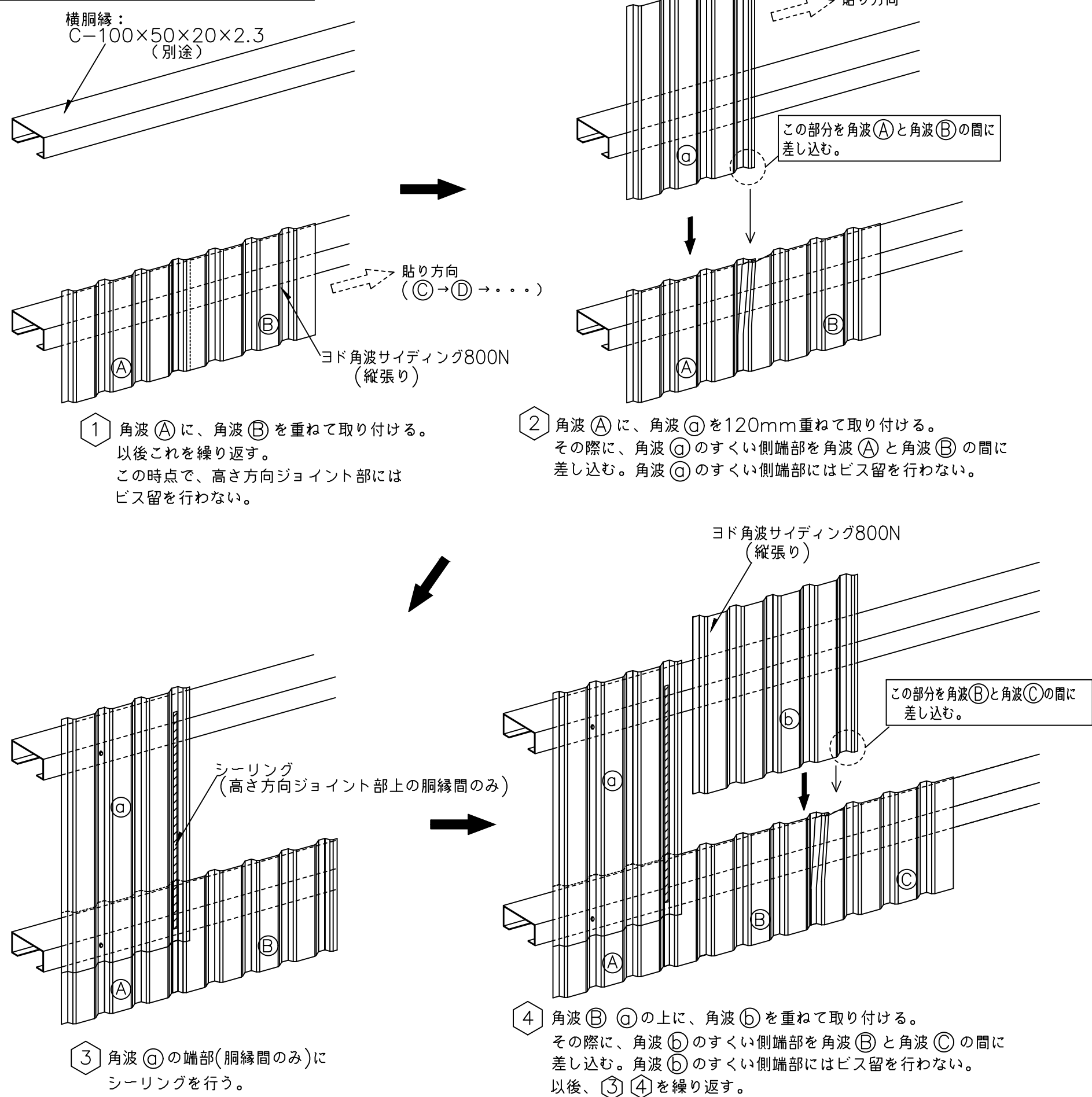
高さ方向ジョイント部 重ね手順図
