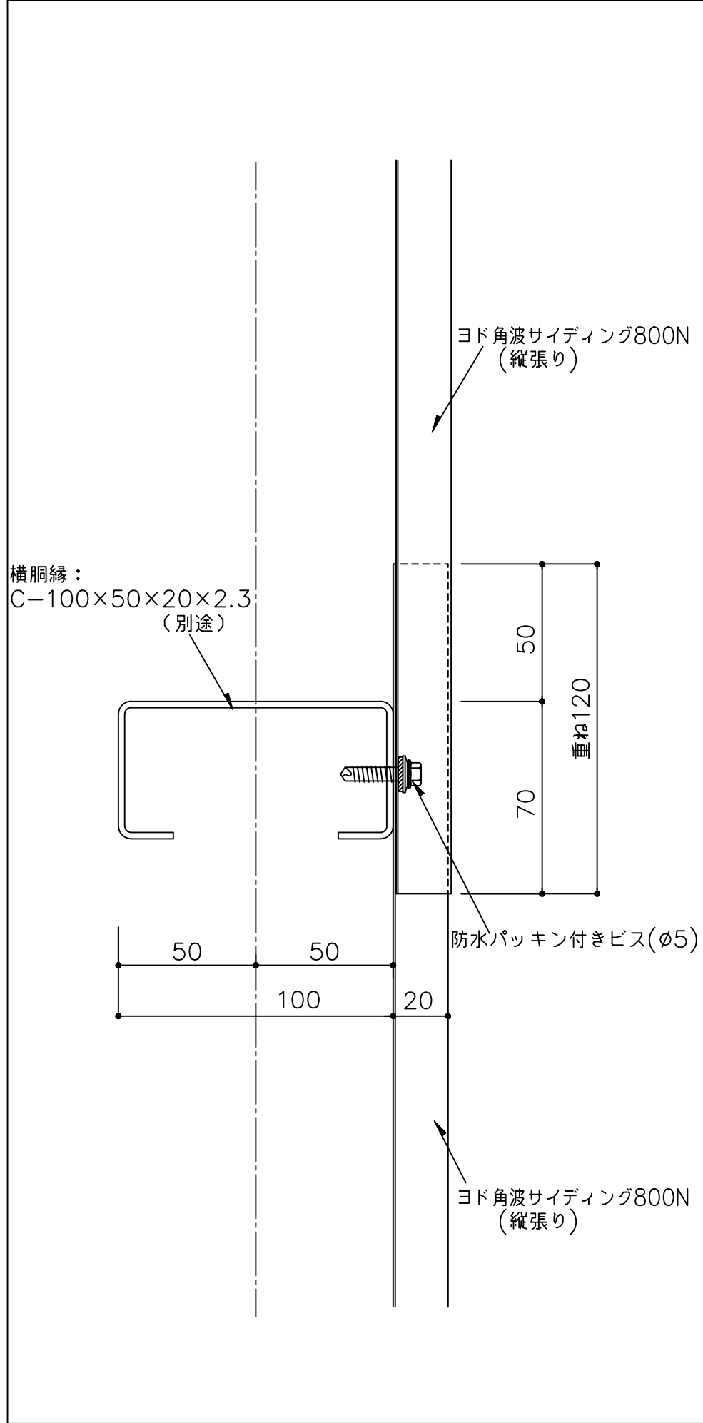
高さ方向ジョイント部 重ね手順図
