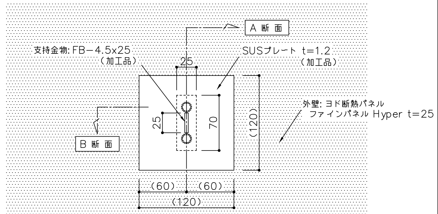
C 立面
