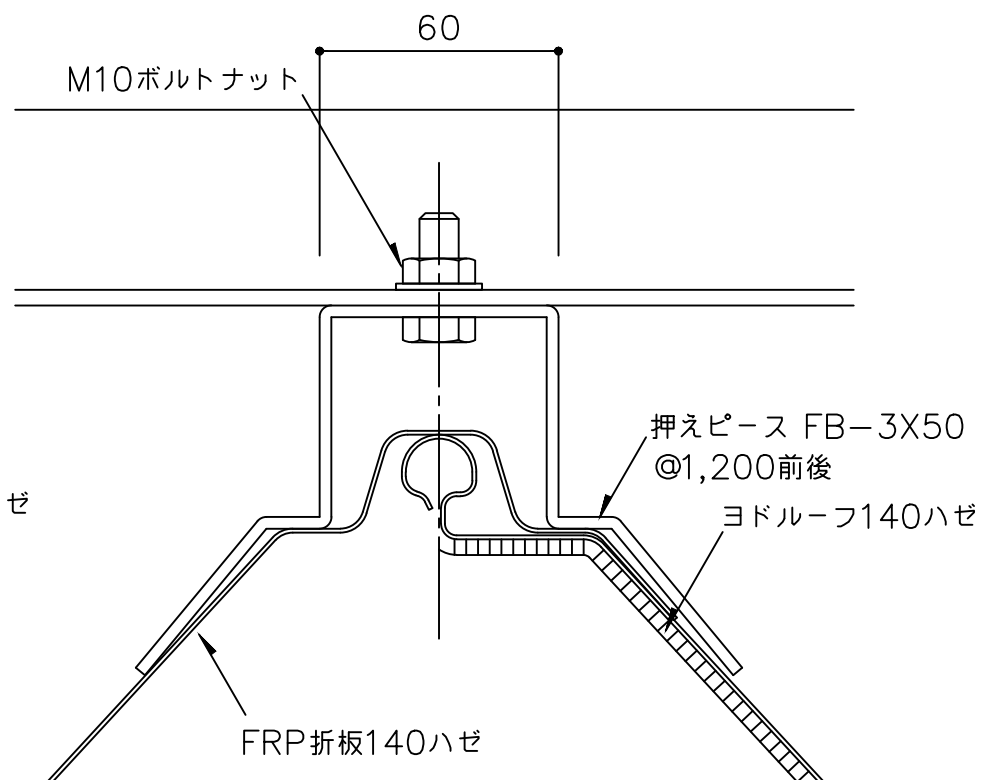
B 詳細図 1/2
