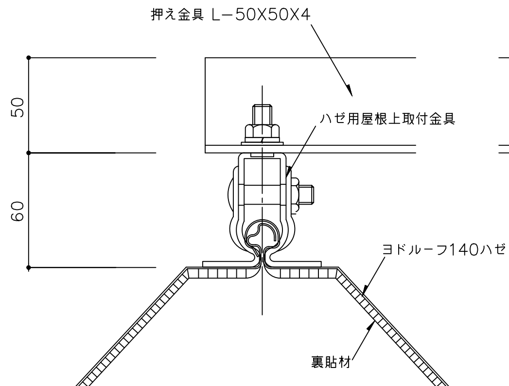
A 詳細図 1/2
