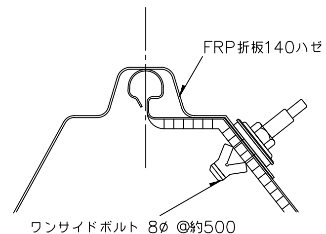
B' 中間部 詳細図 1/2
